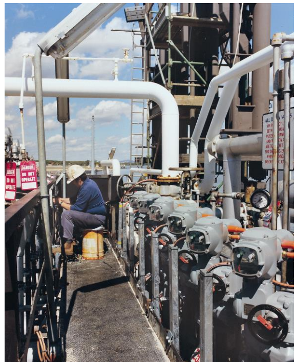
FOTO A: Batteria di valvole motorizzate con attuatori AUMA Matic in versione Profibus.
