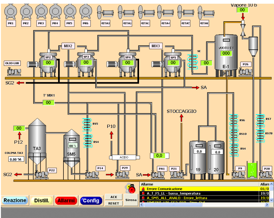
La parte dei reattori nella quale si gestisce la Centrifugazione. Grazie alla supervisione intuitiva, si migliora la produttività.
