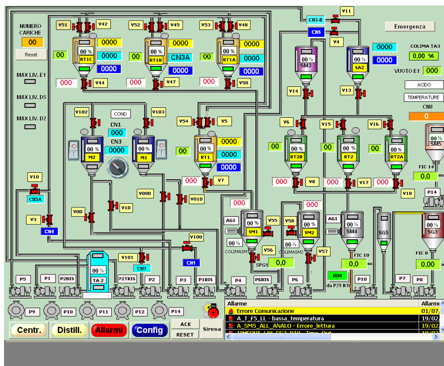
Visualizzazione grafica di uno degli impianti di reazione.
