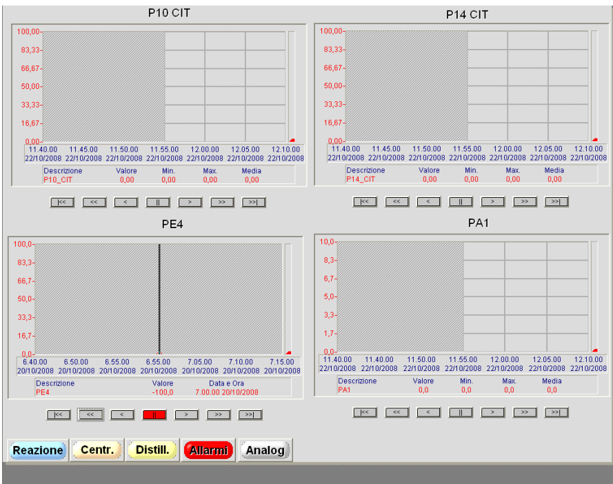
Esempi di visualizzazione grafica delle grandezza analogiche, che possono avvenire sia in tempo reale che su analisi storica.
